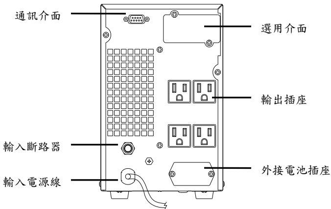
↑ 圖1-1 C-1000F(S)後蓋板
