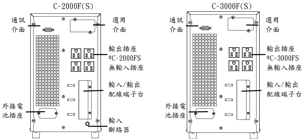
↑ 圖 1-2 C-2000F(S)、C-3000F(S)後蓋板
