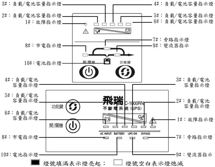
↑圖3-1 操作顯示面板燈號說明
